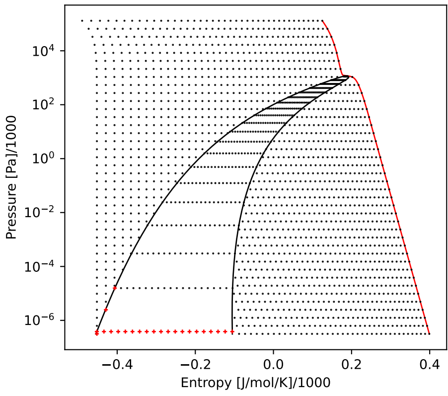
DmolarP
