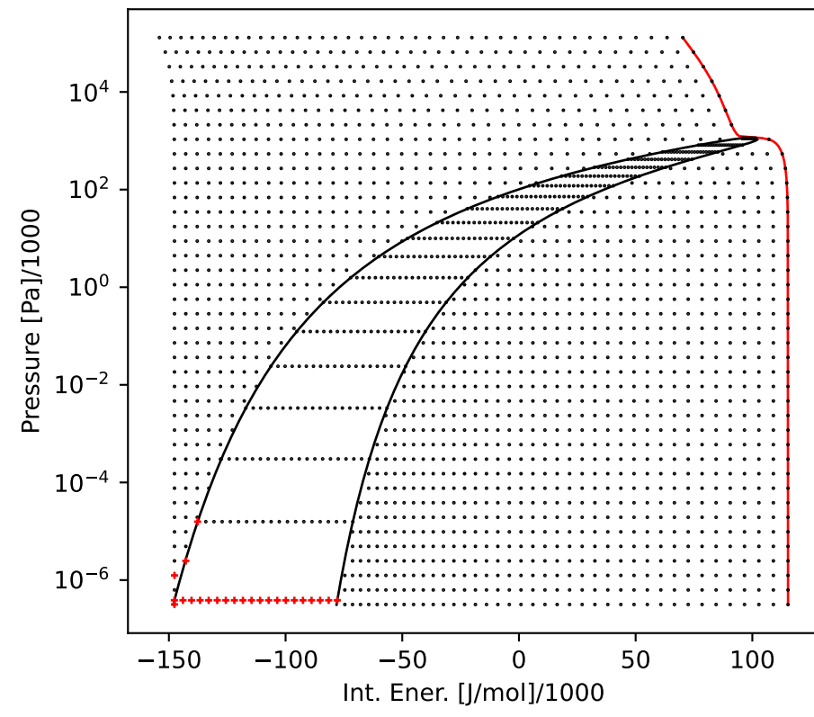
DmolarSmolar
