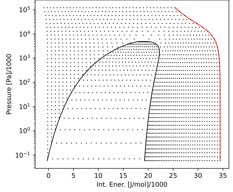
DmolarSmolar
