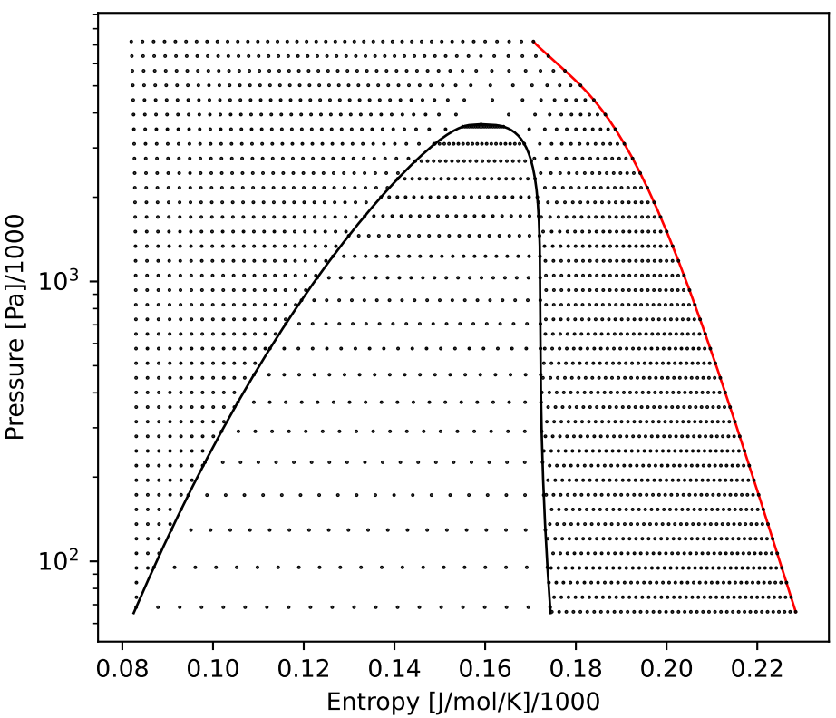
DmolarP
