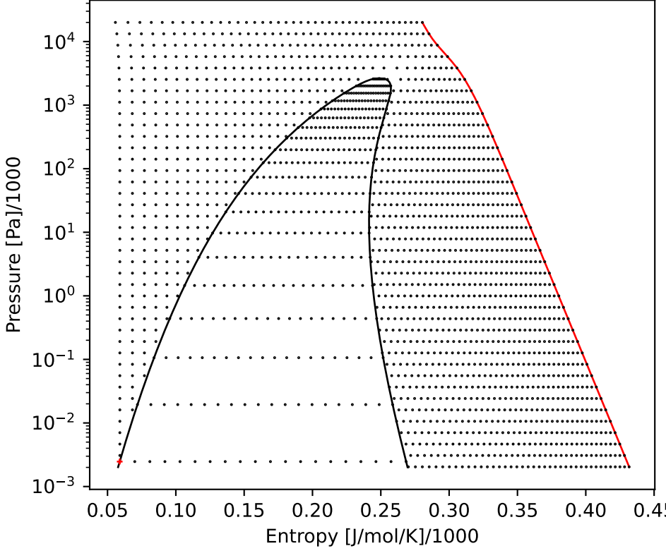
DmolarP
