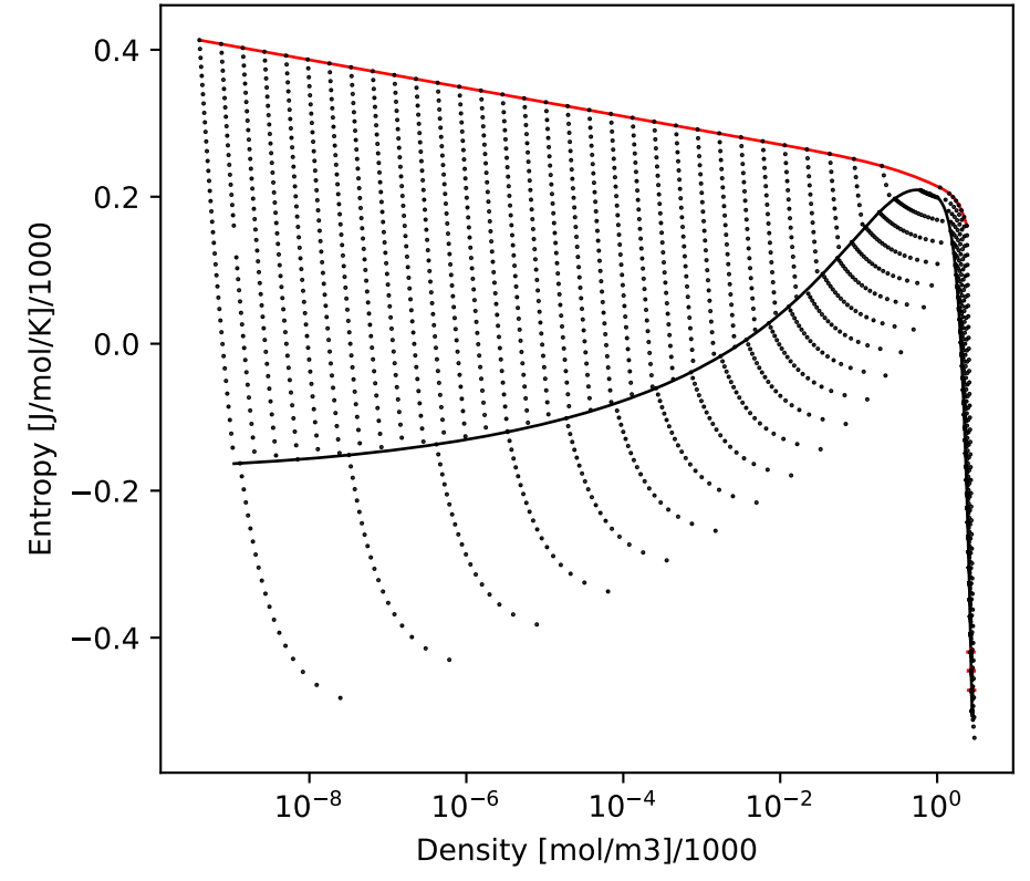
HmolarT
